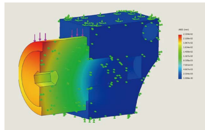
Bewertung der Antriebseinheit für das Hochvakuum-Transferventil (Spannungsanalyse)
